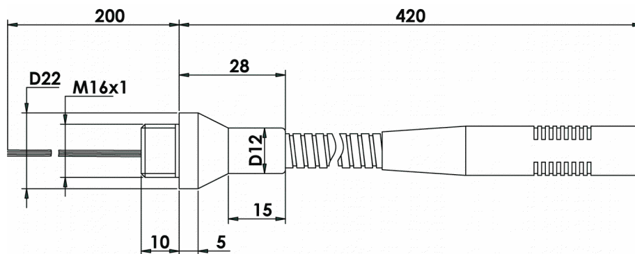
Габаритный чертеж
